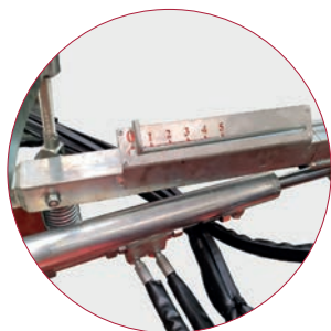
Tastatore a molla regolabile con pistone idraulico Adjustable spring feeler with hydraulic piston Einstellbarer federfühler mit hydraulikkolben Palpeur à ressort réglable avec piston hydraulique Palpador de muelle regulable con pistón hidráulico
